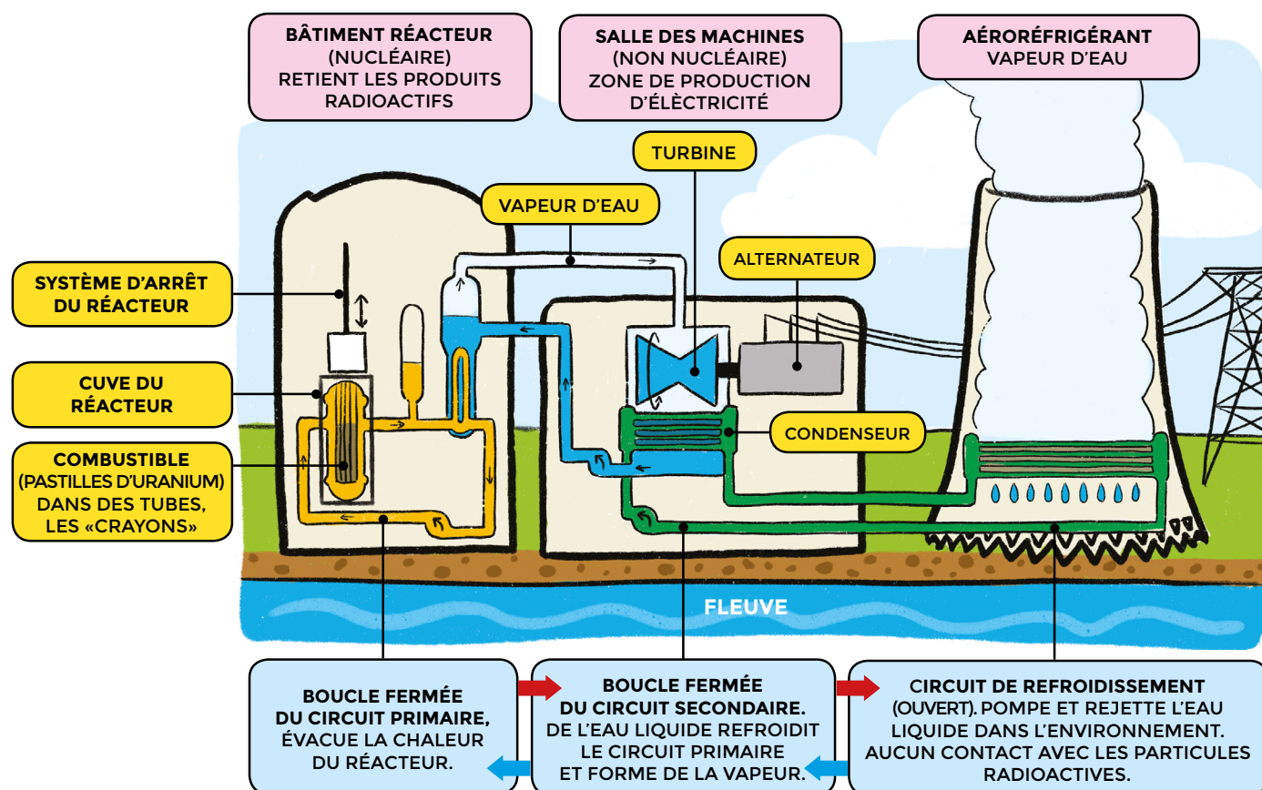
Figure 1 - Fonctionnement d'une centrale nucléaire au bord d'un fleuve (extrait de l'exposition ASN/IRSN)
